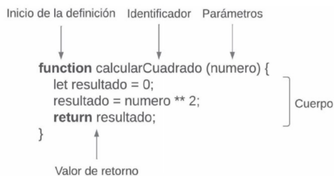
Figura 4.1. Diagrama con los elementos constitutivos de una función en notación declarativa.
